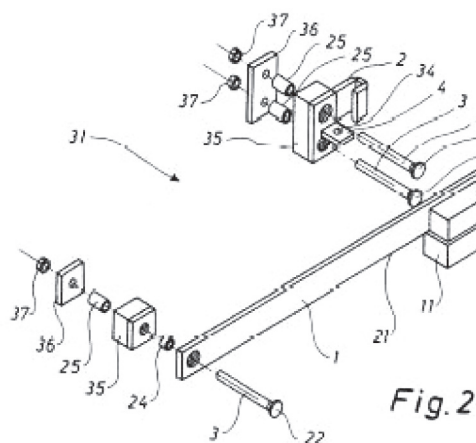
Sprængbillede af den patenterede låseboom.
