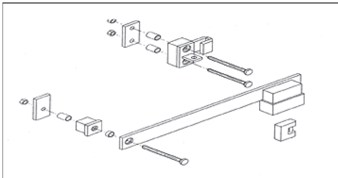
Sprængbillede af kopilåsebom.
